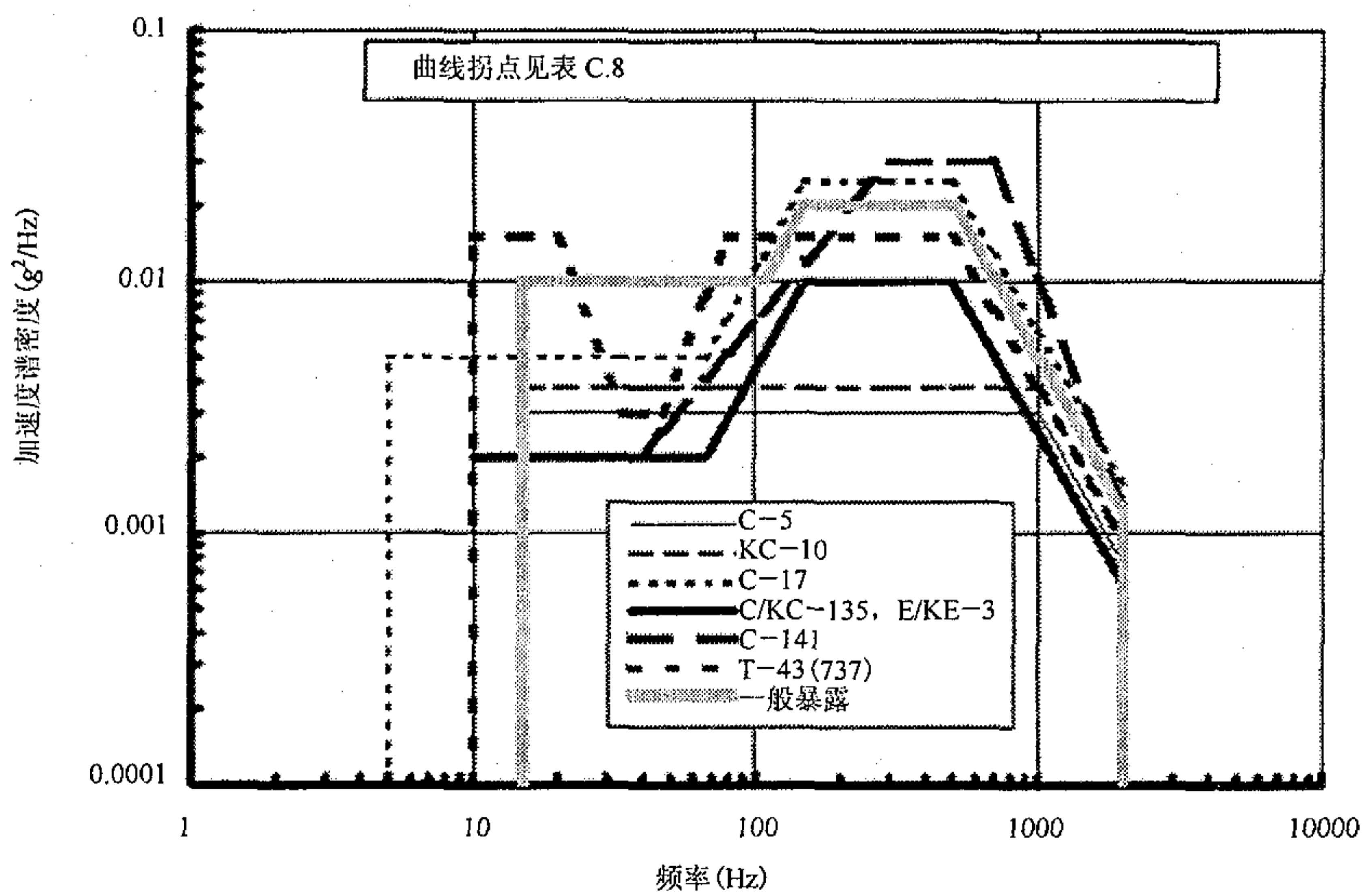
图 C.6 喷气式飞机货物振动环境
